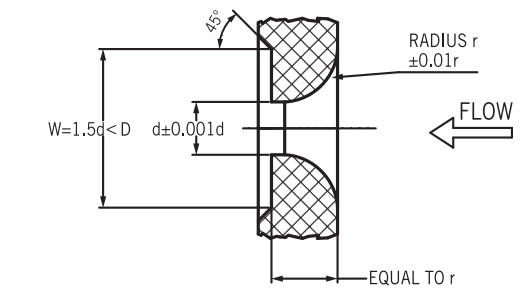
Quadrant Edge Orifice Plate
