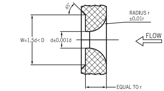
Quadrant Edge Orifice Plate
