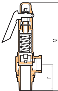
N9LSP TYPE Lever 1/2"~2"
