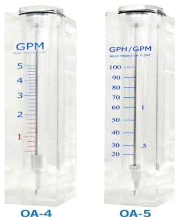
Đồng hồ lưu lượng OA series
