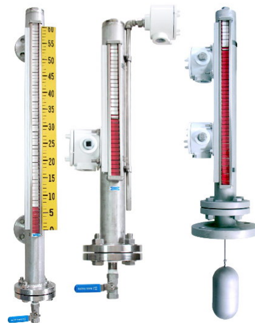
Thiết bị đo mức, báo mức M-series
